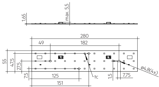
LLE 55x280mm 2000lm LV ADV5
