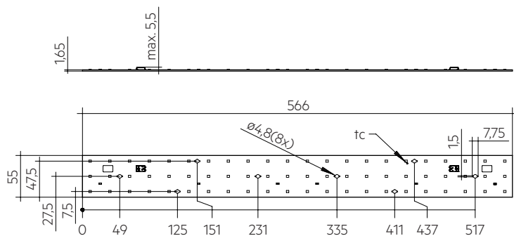
LLE 55x566mm 4000lm LV ADV5
