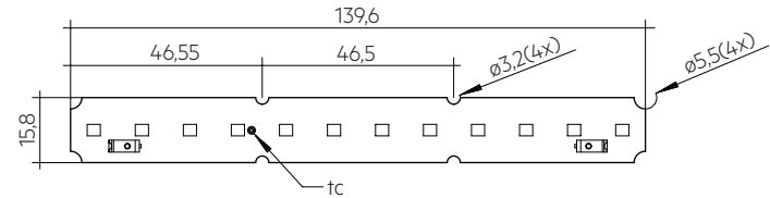
LLE 16x140mm 650lm HV ADV5
