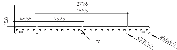
LLE 16x280mm 1250lm HV ADV5
